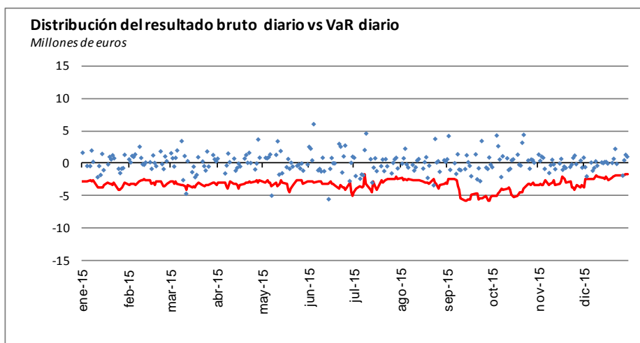
Gráfico 21. BackTesting bruto
